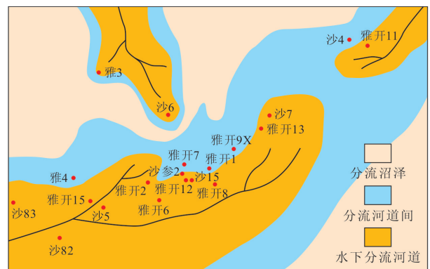
图4 雅克拉断凸下侏罗统4砂组沉积微相
