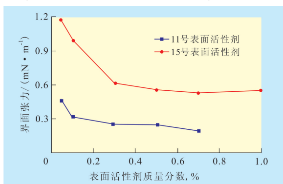
图1 表面活性剂质量分数及与煤油间界面张力的关系
