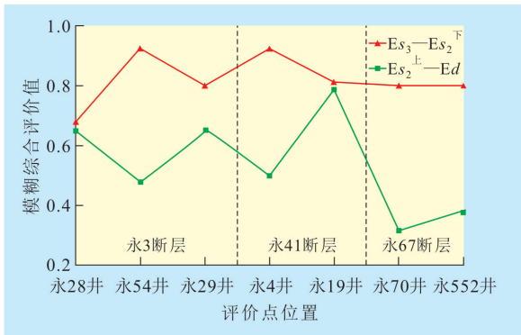
图3 永安镇地区主干断层封闭性模糊综合评价
