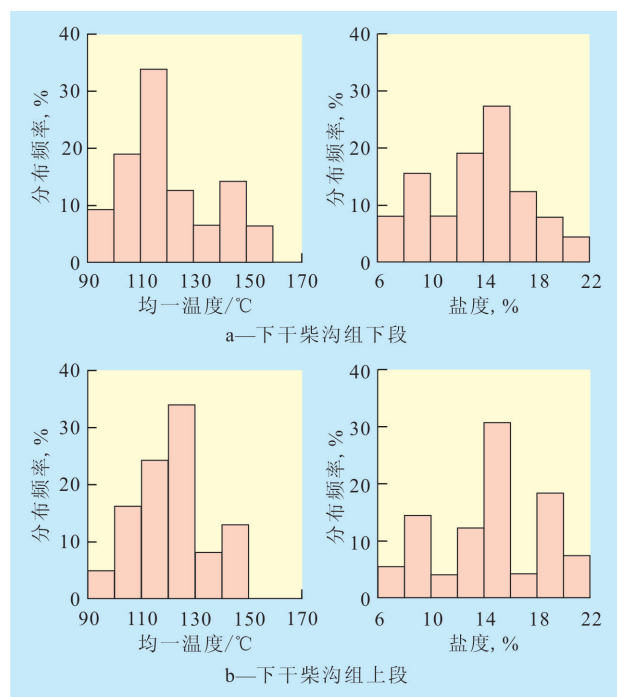
图3 狮子沟油田下干柴沟组储层流体包裹体均一温度和盐度分布
