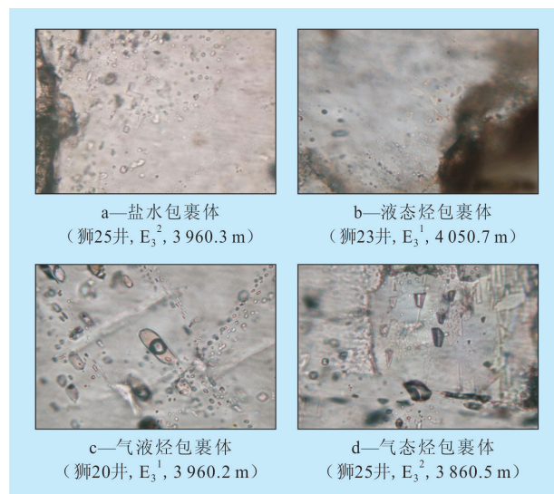
图2 狮子沟油田下干柴沟组储层流体包裹体类型
