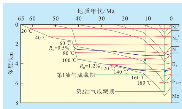
图4 狮子沟油田下干柴沟组油气成藏期次划分
