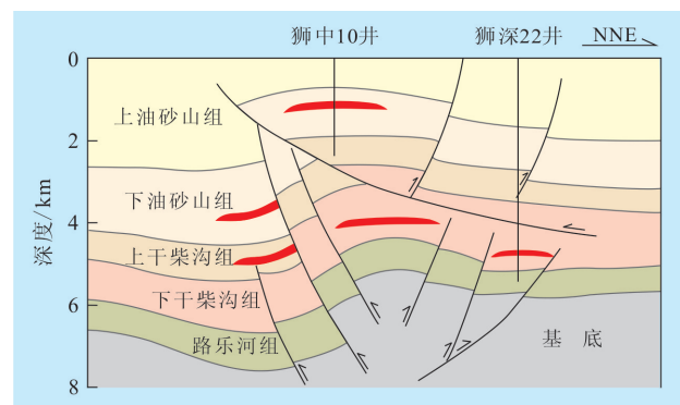
图1 狮子沟油田98SZG测线构造剖面
