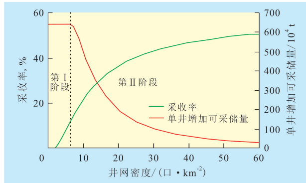
图2 修正后采收率和单井增加可采储量与井网密度的关系
