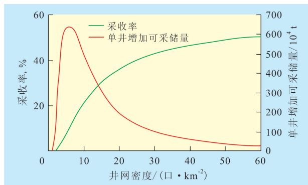
图1 采收率和单井增加可采储量与井网密度的关系
